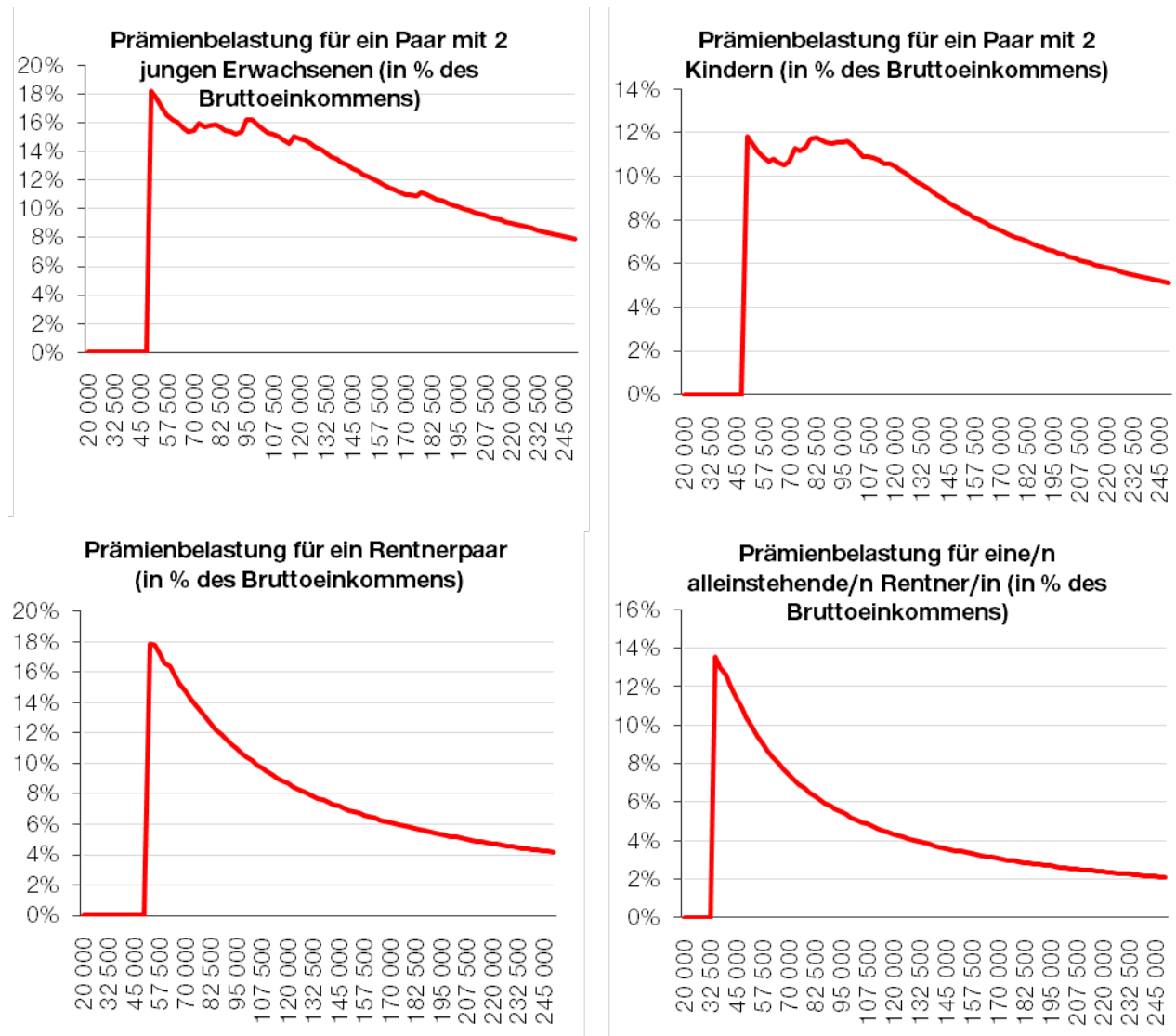
Grafik 9 USS-Berechnung (2018)
